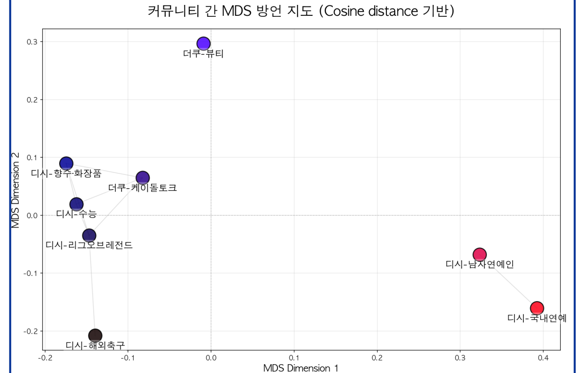
[그림 7] Cosine distance 기반 커뮤니티 간 MDS 방언 지도
